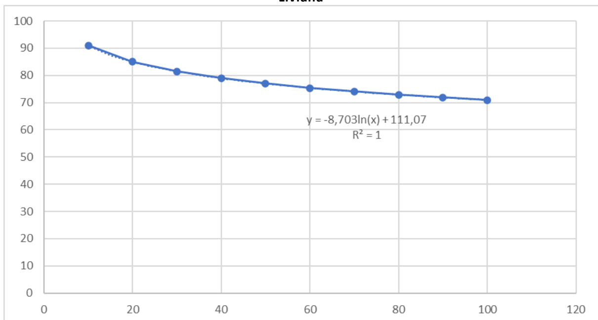
Gráfico 9.2-2: Estimación atenuación geométrica sonido de Equipos y Maquinaria Industrial Liviana
