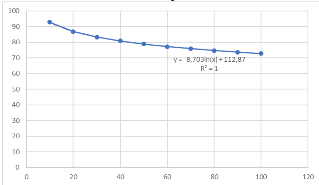
Gráfico 9.2-1: Estimación atenuación geométrica sonido vías de acceso
