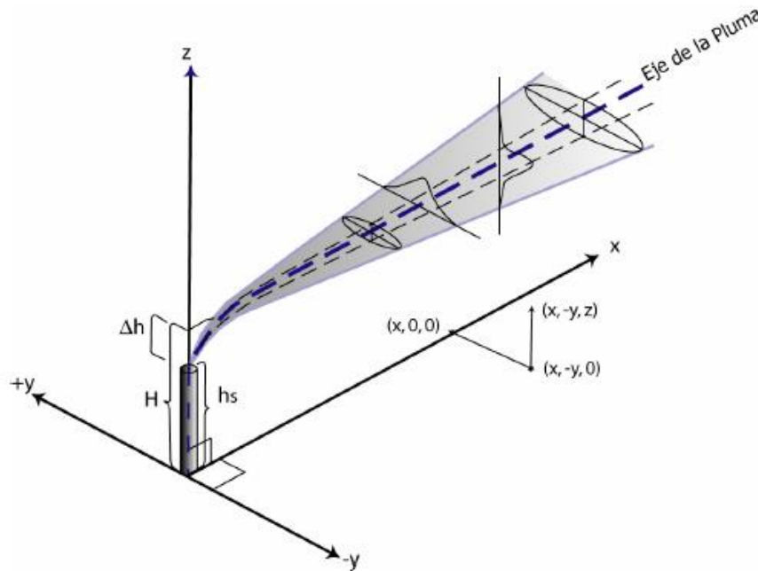
Figura 9.2-1: Columna de humo gaussiana
