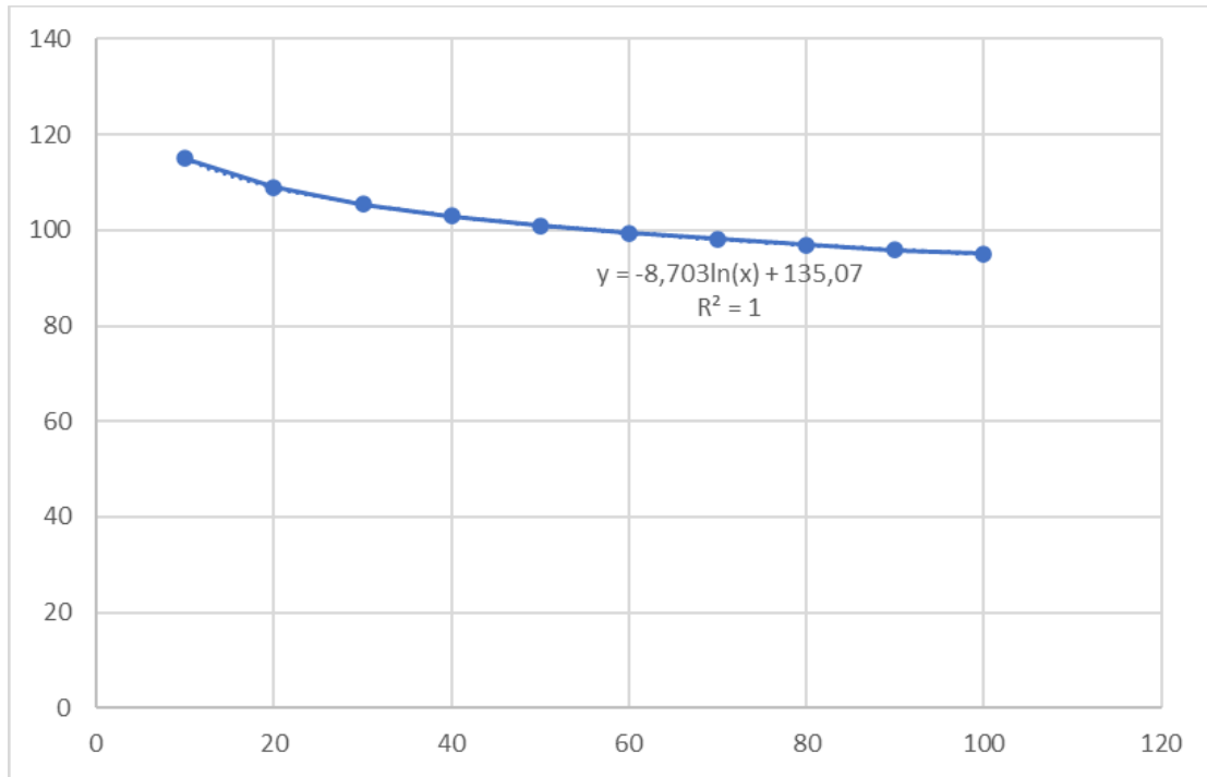
Gráfico 9.2-3: Estimación atenuación geométrica sonido de Equipos y Maquinaria Industrial Pesada
